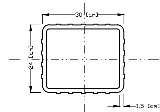
Przekrój profilu z jakiego wykonano drabinę wewnątrz konstrukcji
