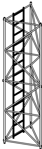
Rzut aksonometryczny segmentu konstrukcji
